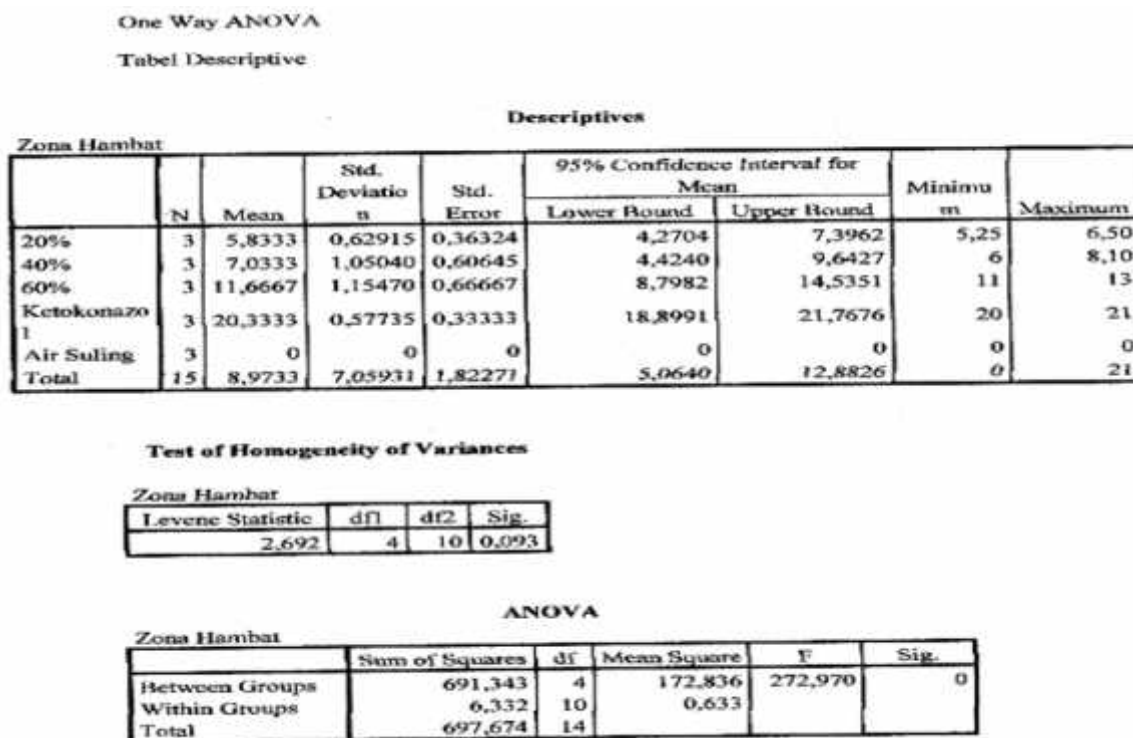
Gambar 2. Gambar descriptive dari one way ANOVA pada perbedaan konsentrasi perlakuan.
