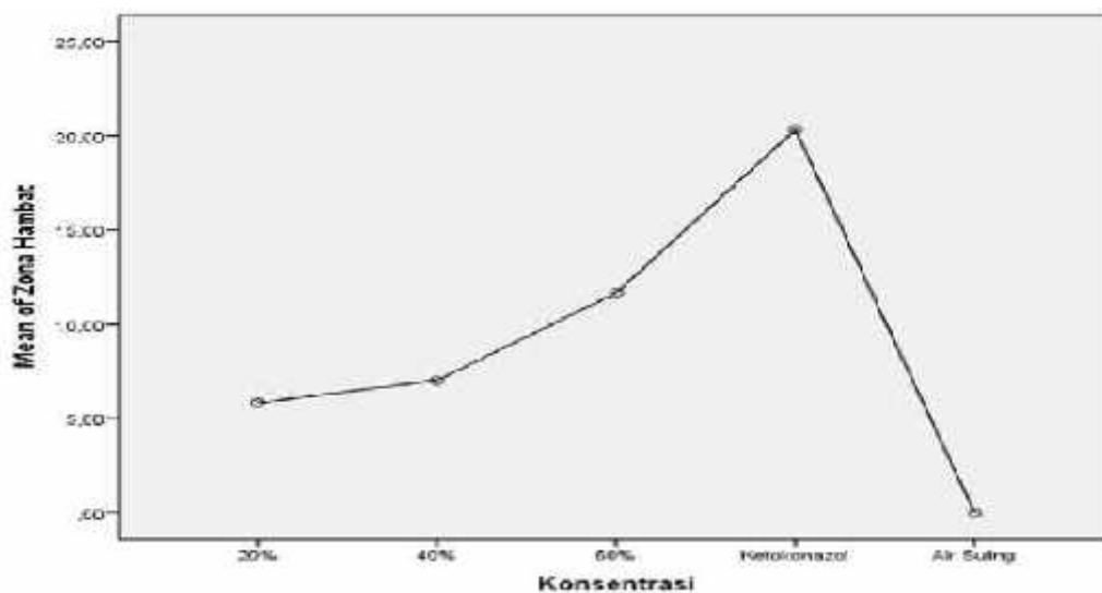
Gambar 2. Gambar descriptive dari one way ANOVA pada perbedaan konsentrasi perlakuan.
